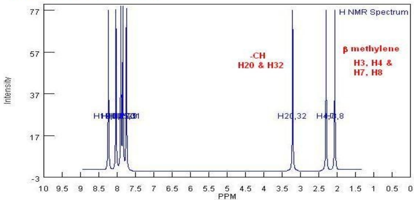
90724_NMR_0to10.jpg
